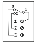
Without midictor Изходни клеми (директно свързване)
